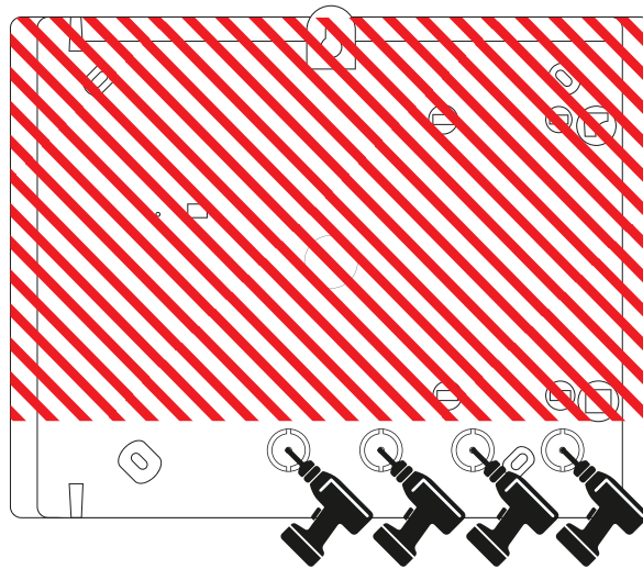
Ansicht Rückseite
