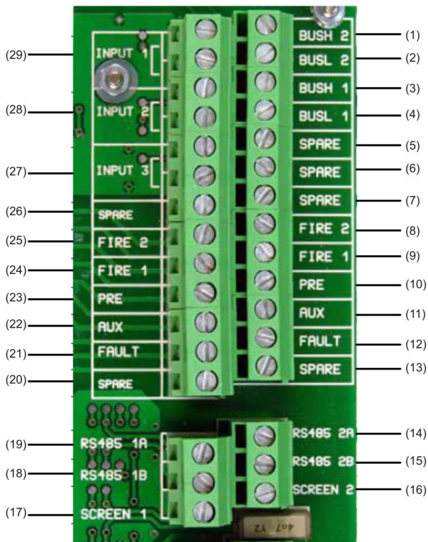
Figura 14: Collegamenti della morsettiera del rivelatore
