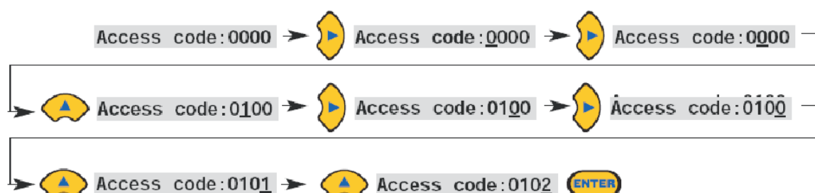
Figura 27: Impostazione del codice di accesso
