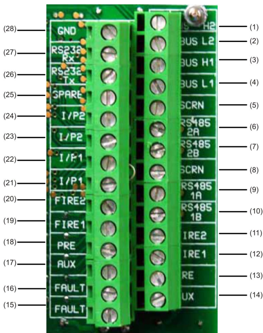
Figura 15: Collegamenti della morsettiiera del modulo di comando
