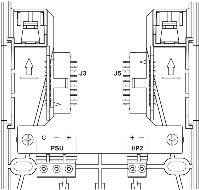
Afbeelding 13: Printplaat aansluitingen van grondplaat (onderzijde)
