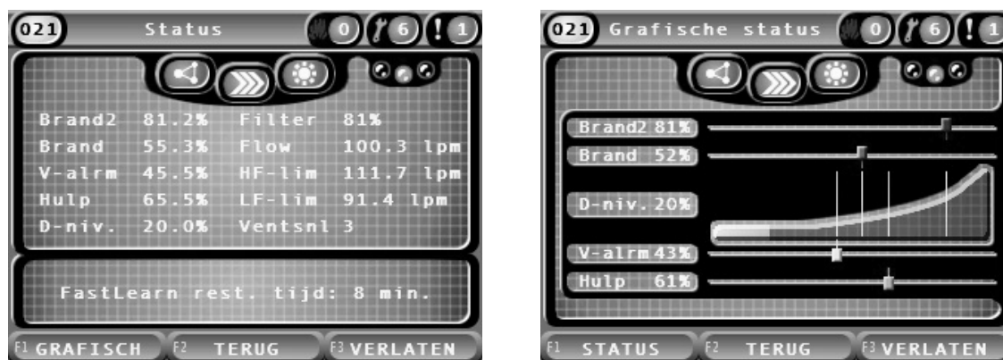
Afbeelding 22: Detectorstatusschermen
