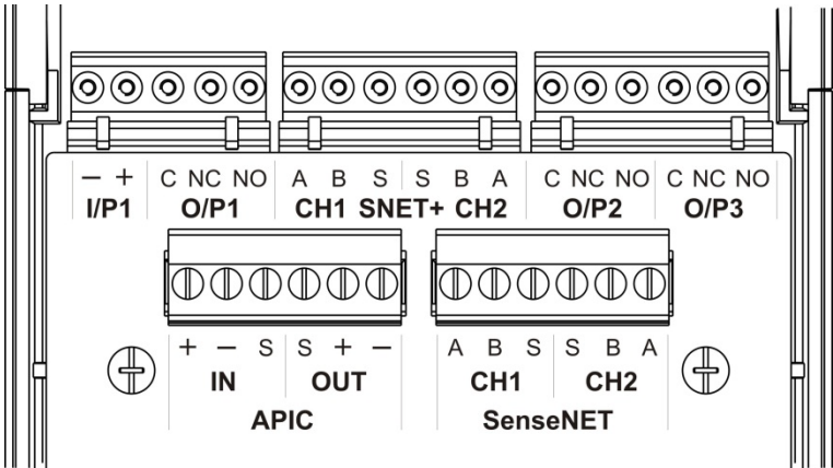
Afbeelding 12: Printplaat aansluitingen van grondplaat (bovenzijde)
