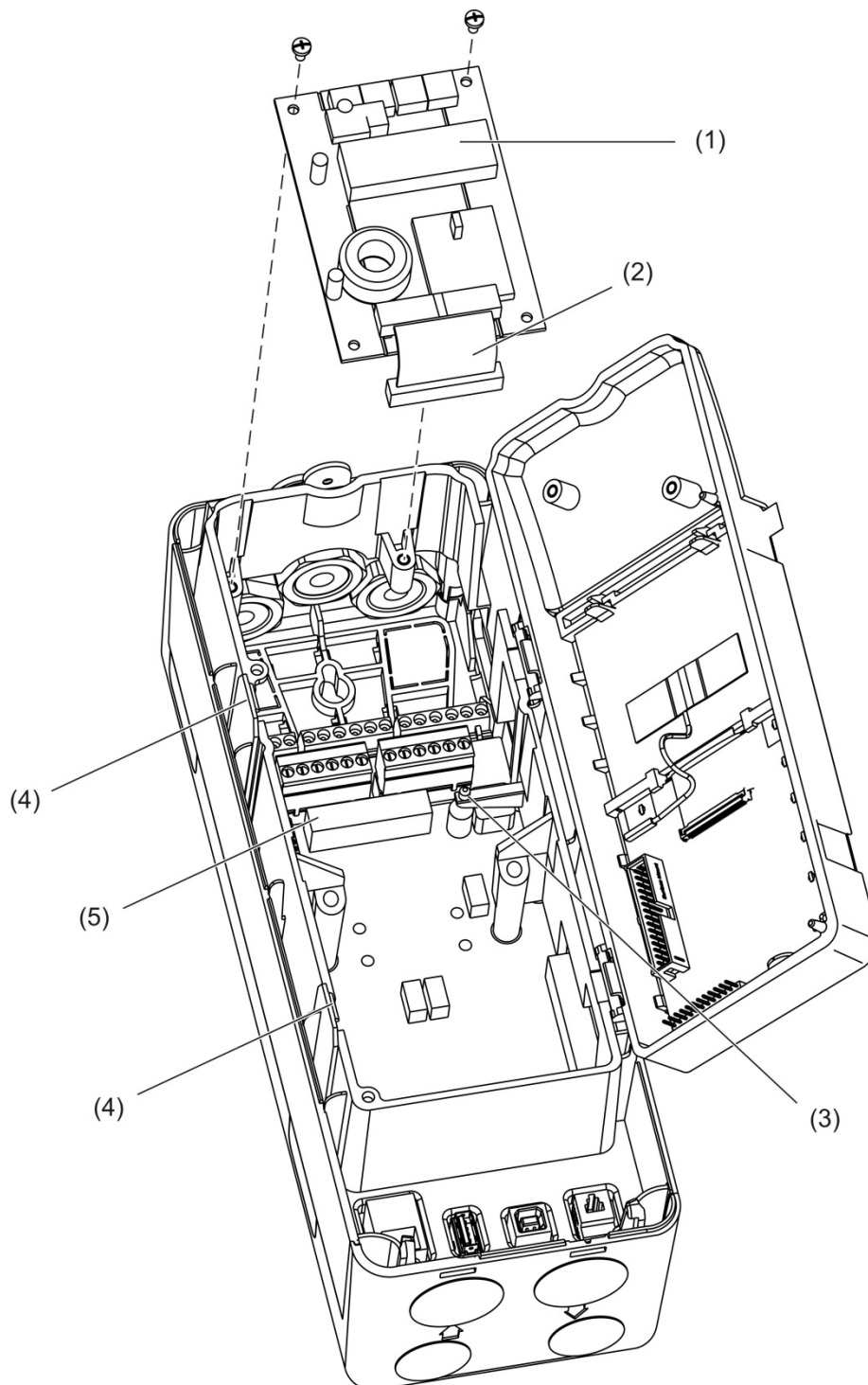
Afbeelding 27: APIC installeren
