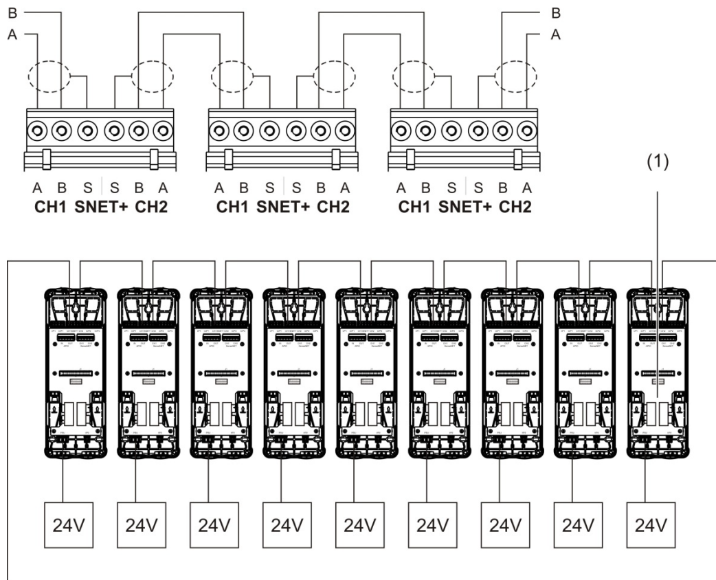
Afbeelding 15: Gedistribueerd cluster
