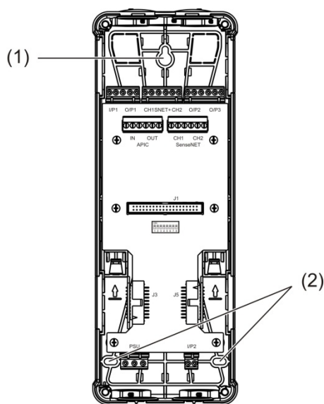
Figura 10: Instalar el panel posterior en una pared
