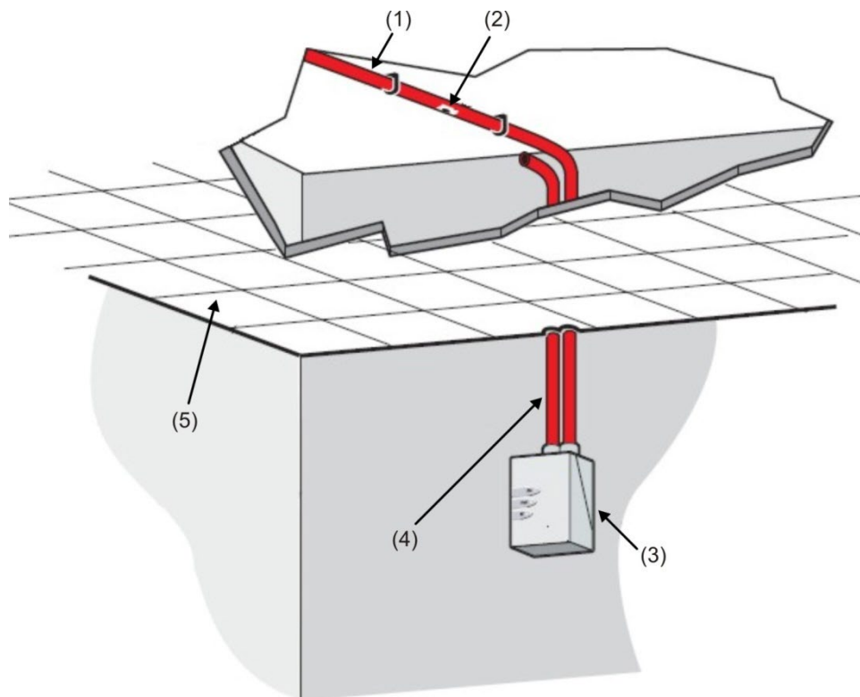
Rysunek 6: Instalacja rur powyżej sufitu podwieszanego z widoczną czujką (z rurą wylotową)
