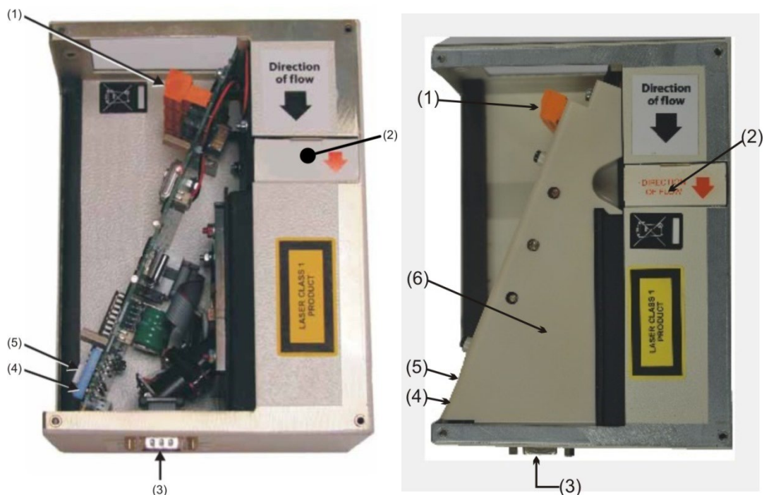
Rysunek 2: Widok wewnętrzny czujki (modele EN / UL)
