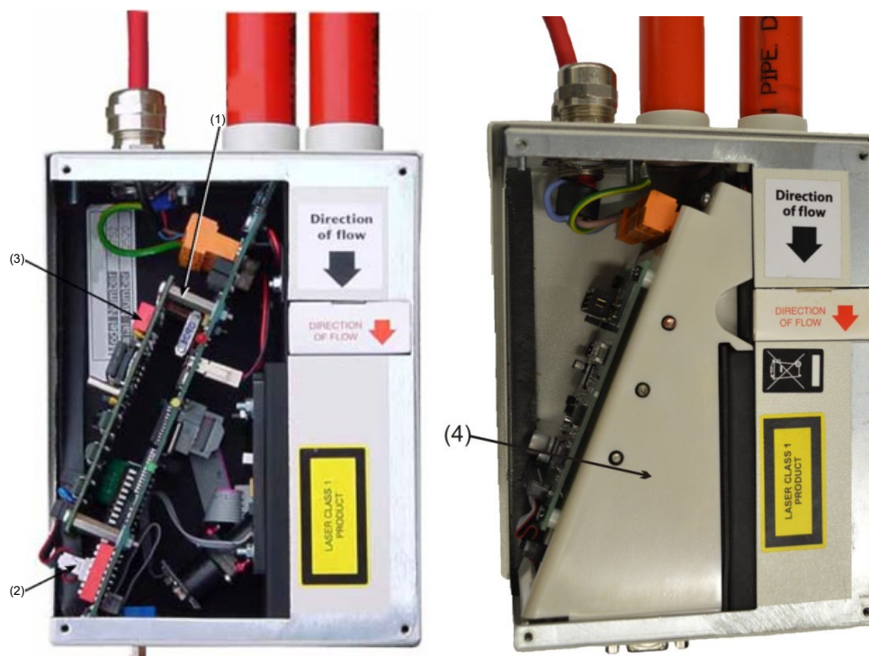
Rysunek 13: Połączenia karty APIC (modele EN / UL)
