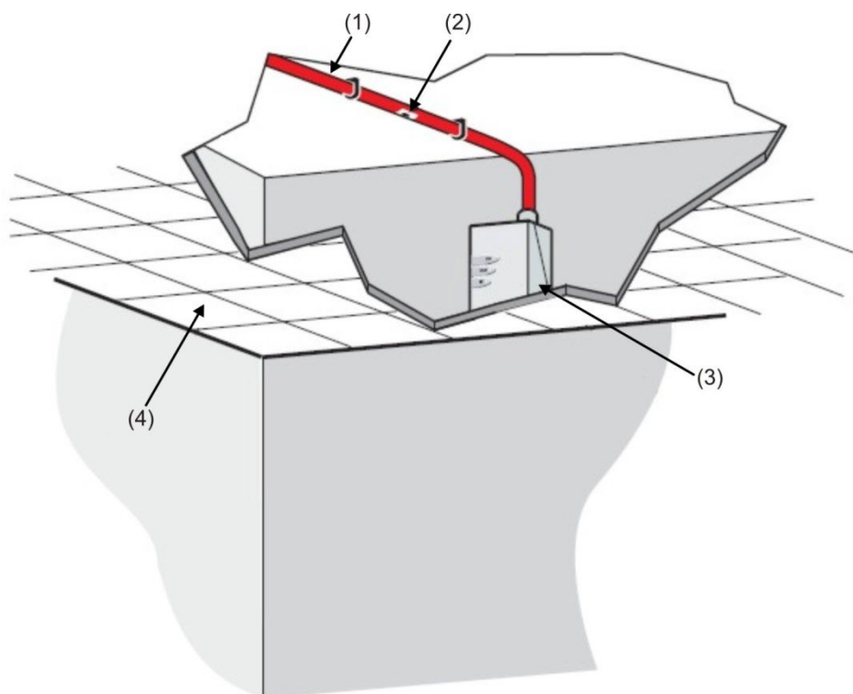
Rysunek 7: Instalacja rur powyżej sufitu podwieszanego z czujką zamontowaną w obszarze międzystropowym (bez rury wylotowej)
