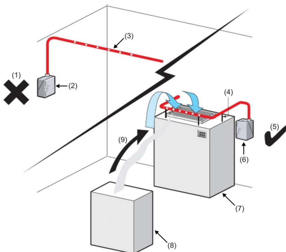
Rysunek 5: Urządzenie wentylacyjne w bezpośredniej bliskości czujki (pokazano wylot w celu zapewnienia przejrzystości)
