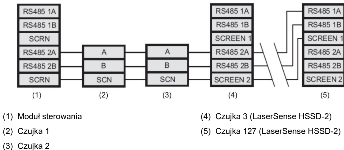
Rysunek 15: Podłączanie czujki do sieci SenseNET
