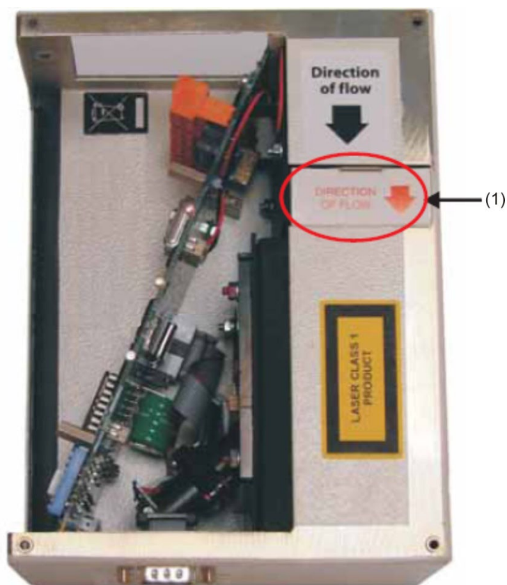
Rysunek 19: Lokalizacja wkładu filtra
