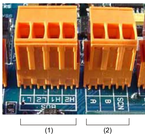
Rysunek 10: Złącza adresu APIC i RS-485/SenseNET
