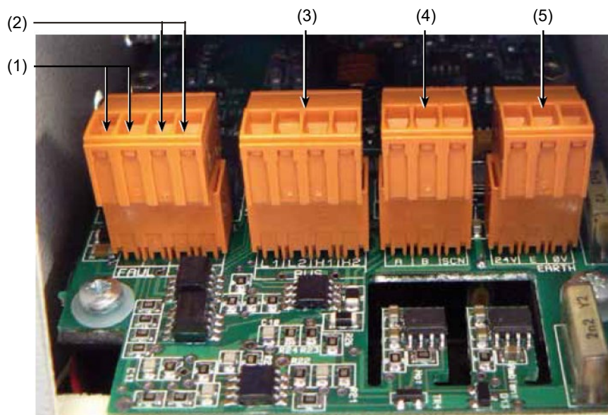
Rysunek 3: Połączenia bloku złączy czujki
