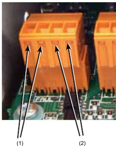
Rysunek 12: Styki przekaźników uszkodzenia i pożaru (alarmu)
