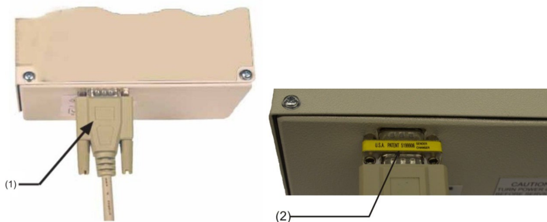
Rysunek 18: Połączenie portu szeregowego czujki do komputera
