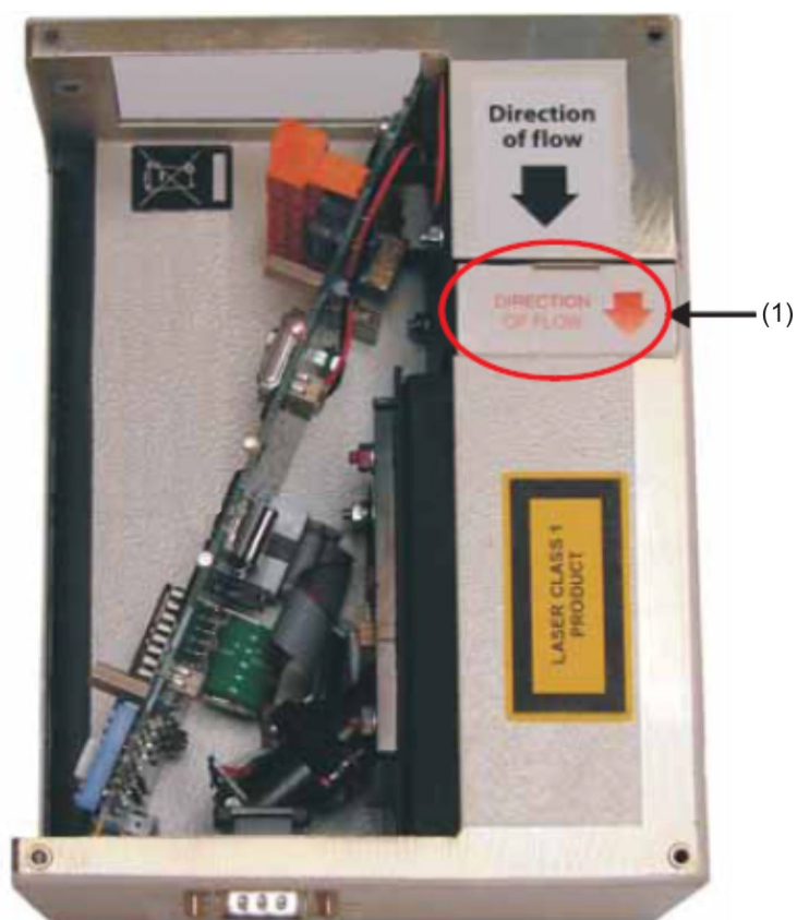
Figura 19: Ubicación del cartucho del separador de polvo
