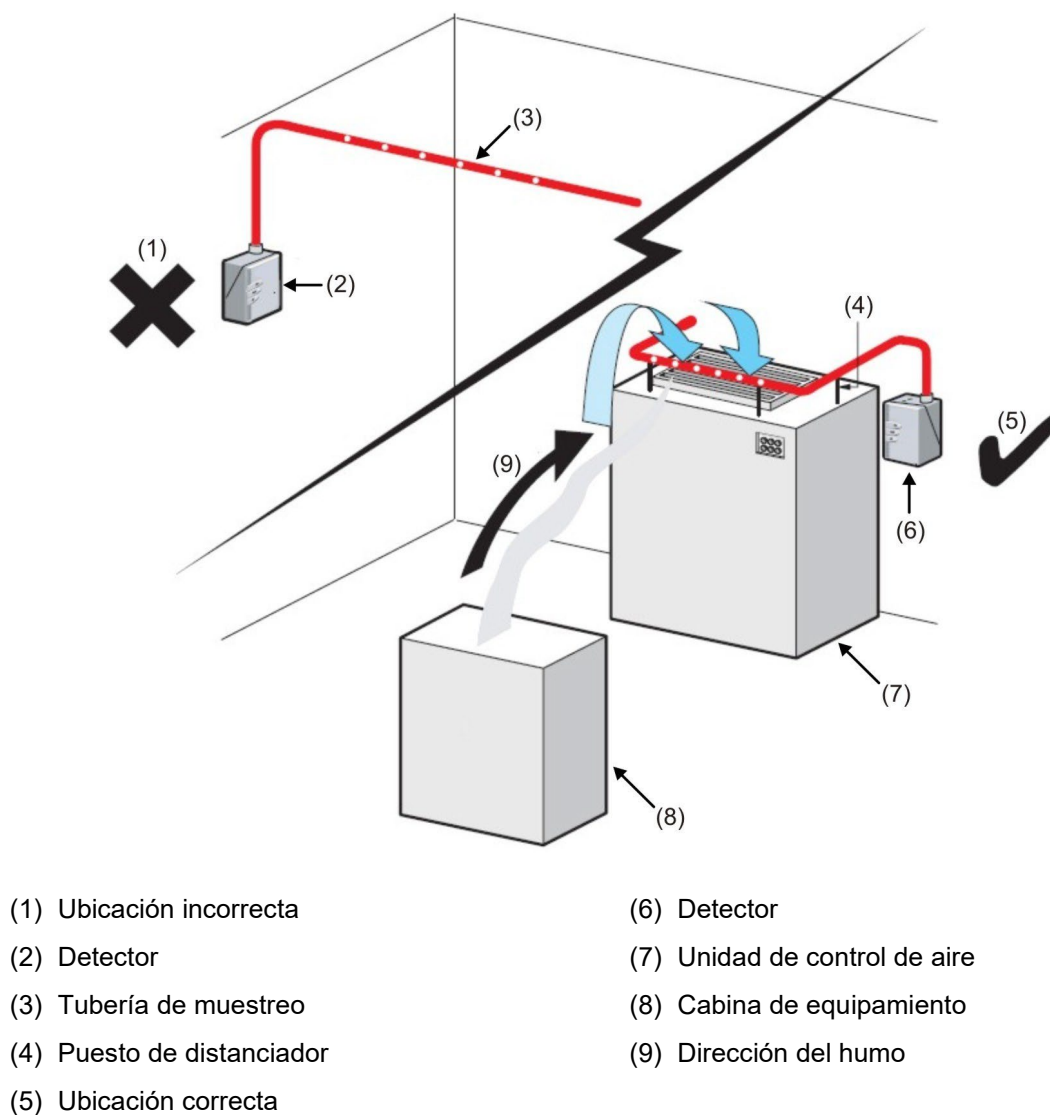
Figura 5: Unidad de control de aire en las proximidades del detector (escape ilustrado para mayor claridad)
