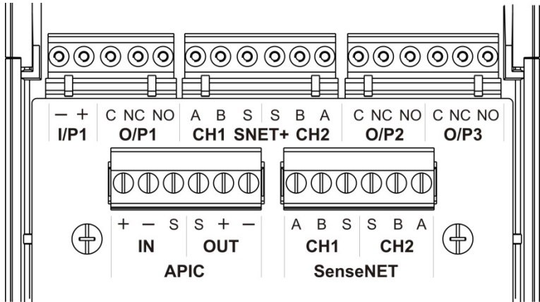
Figura 12: Conectores PCB del panel posterior (parte superior)
