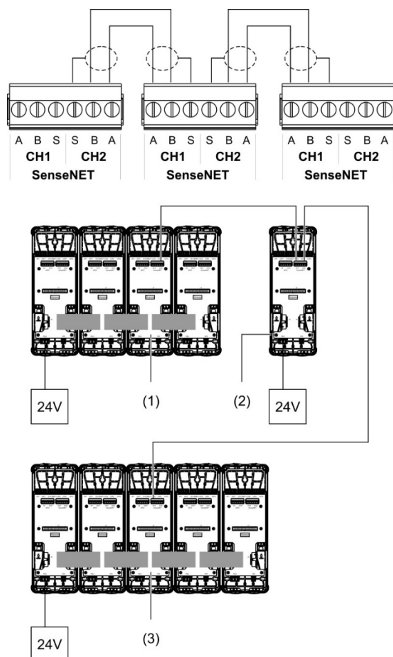
Figura 17: Conectar una red de varios clústeres
