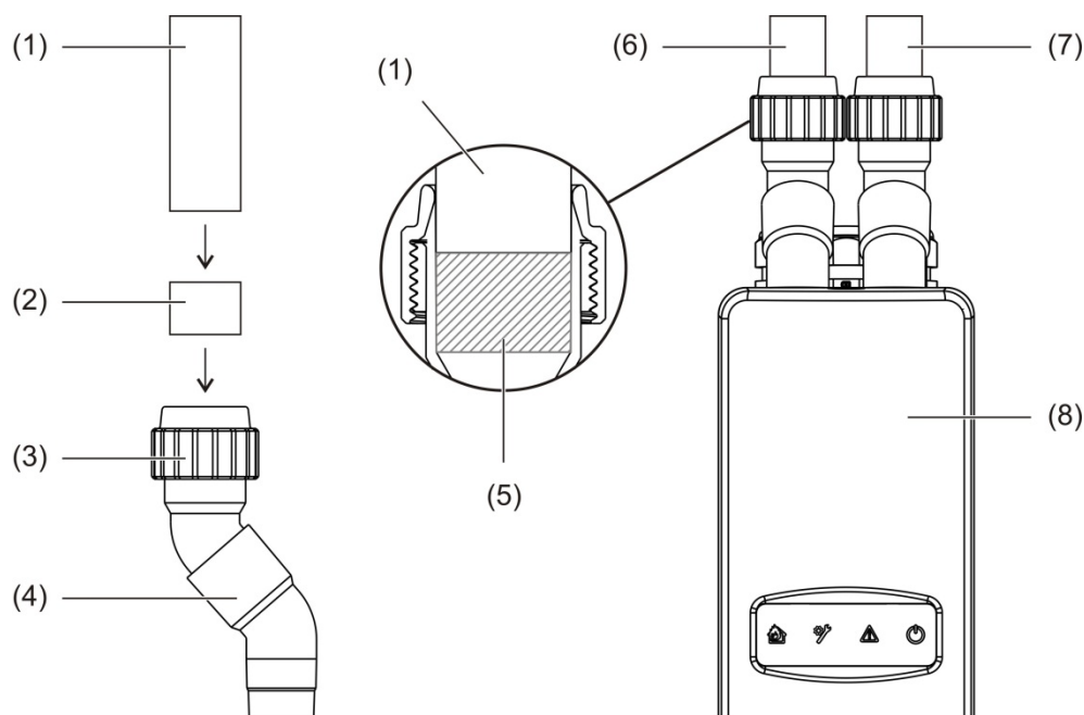
Figura 20: Conexión de tuberías mediante un adaptador de tuberías
