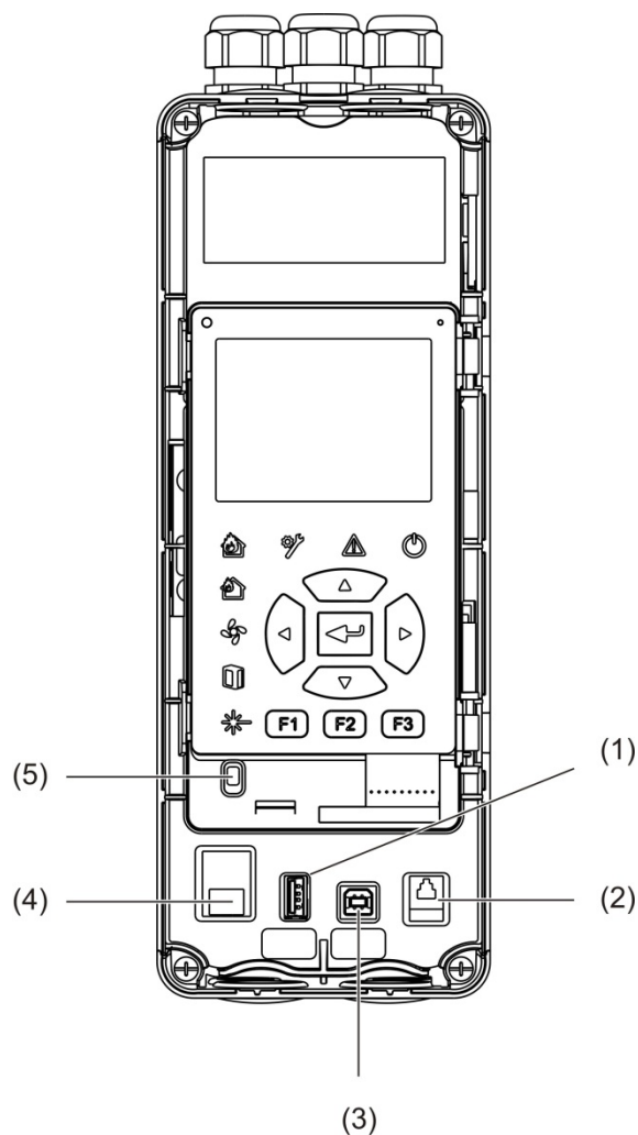
Figura 7: Diagrama del módulo de visualización
