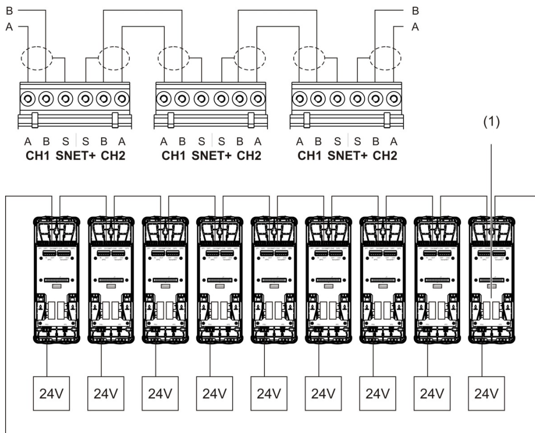
Figura 15: Clúster distribuido
