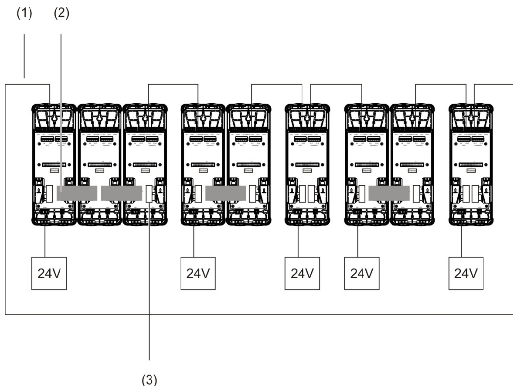
Figura 16: Clúster híbrido
