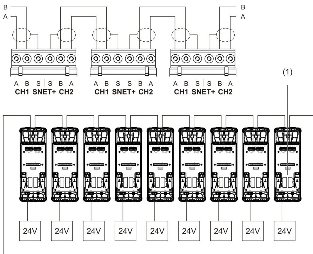
Figure 15 : Cluster distribué
