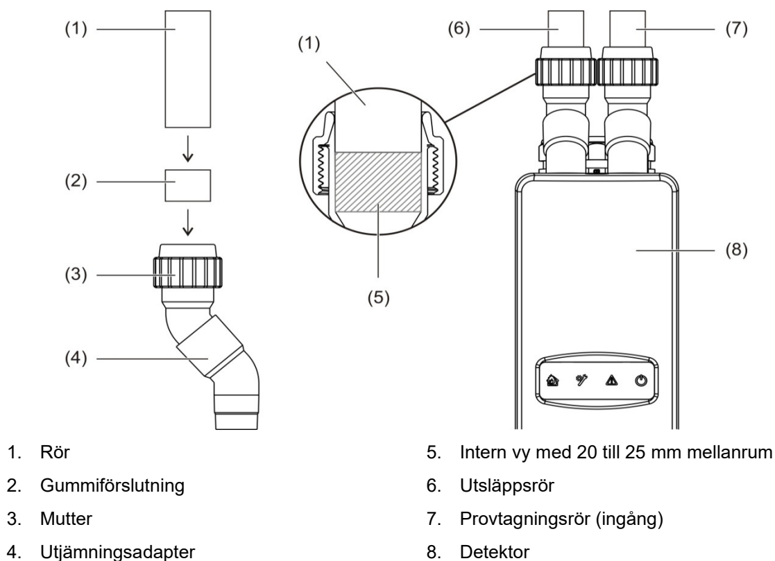
Bild 20: Ansluta rör med hjälp av en röradapter
